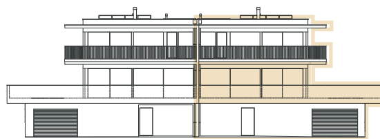
FAÇADE SUD
